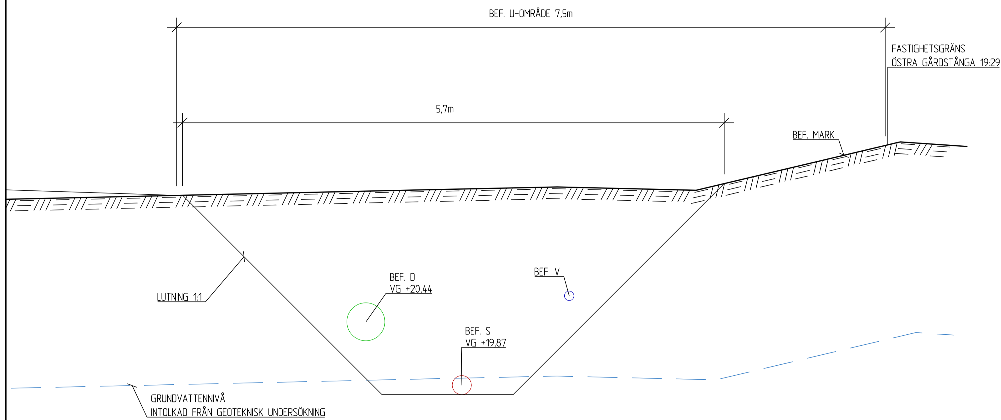
SEKTION C-C SKALA 1:25
